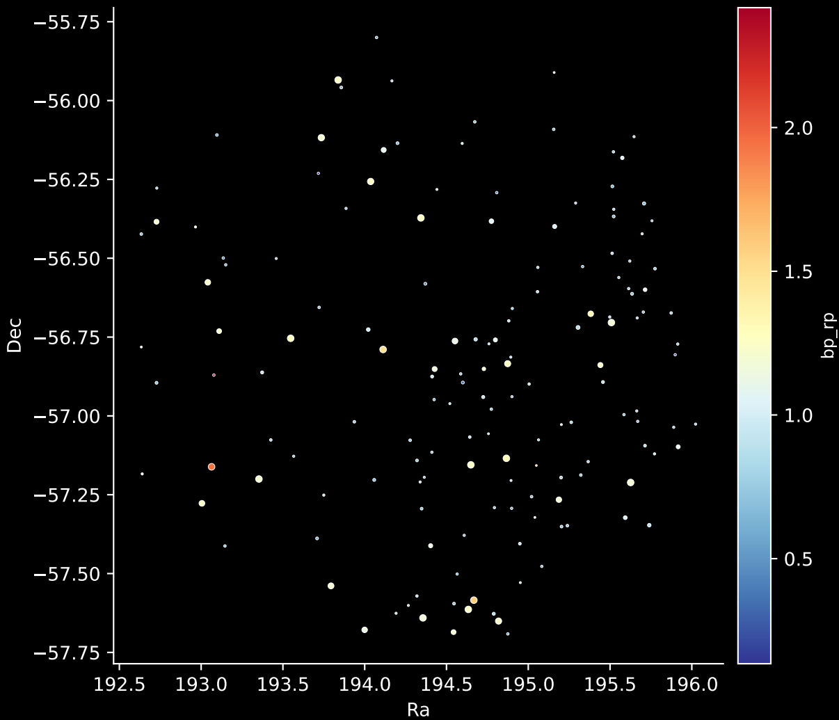
GALAH DR4 Field: [7188] Stars: 154
