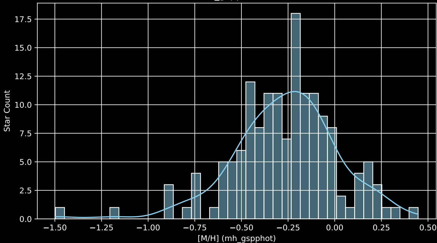
GALAH DR4 Field: [7188] [M/H] (mh_gspphot) (n= 151)
