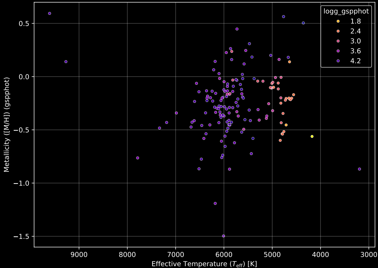
GALAH DR4 Field: [7188] Stellar Population Parameters (n= 154)
