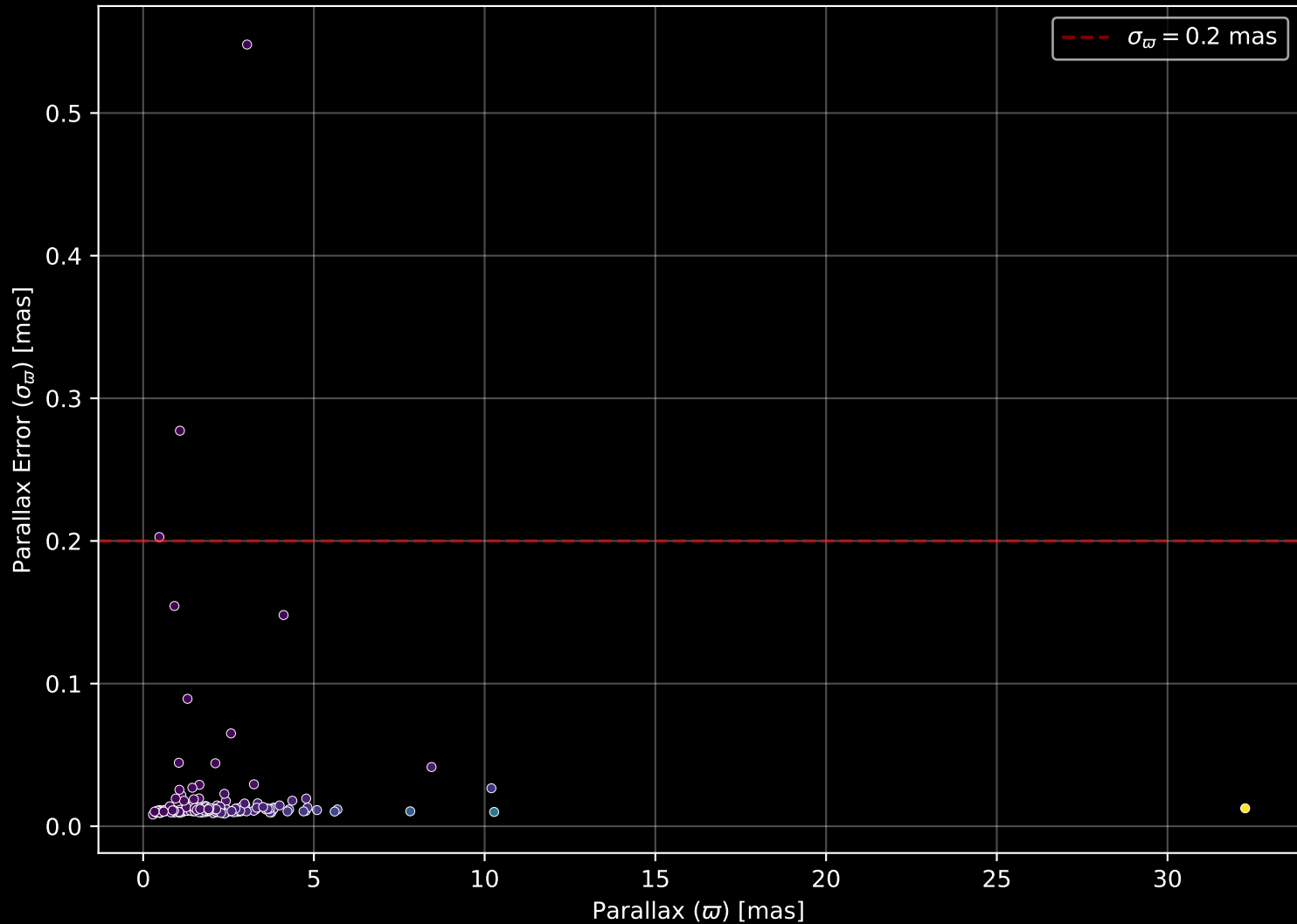
GALAH DR4 Field: [7188] Parallax Quality (n= 154)
